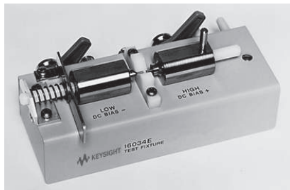
16034E SMD/chip test fixture
